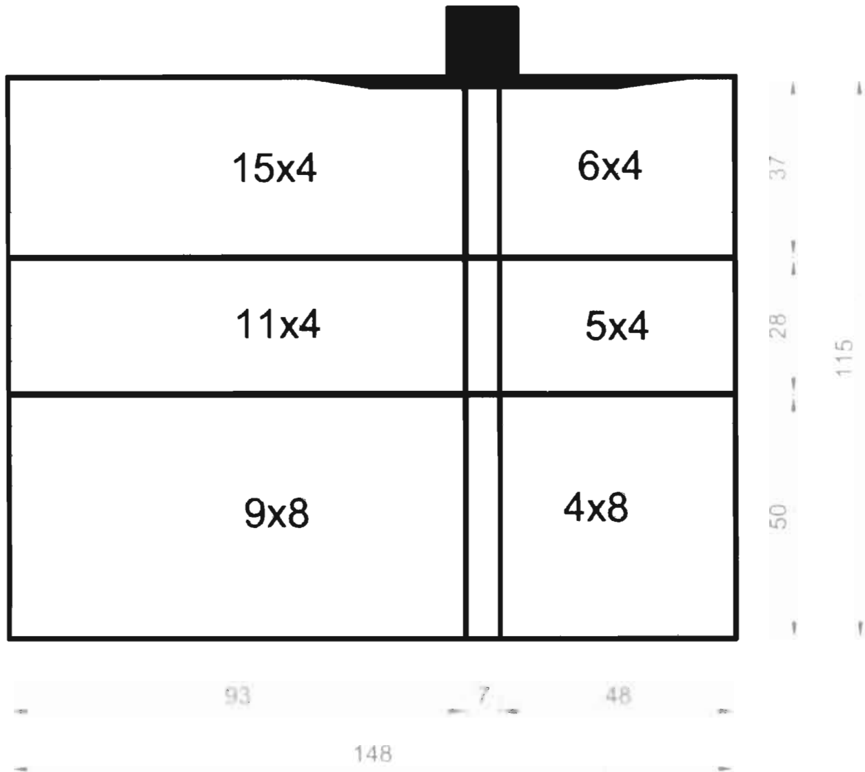
Figura 3. Schema de împărțire în domenii a electrodului. Sunt indicate dimensiunile domeniilor (în milimetri) respectiv numărul de peleti aflați în fiecare dintre aceștia. Distribuția nervurilor care formează peleți în fiecare zonă este uniformă, atât pe orizontală cât și pe verticală.
