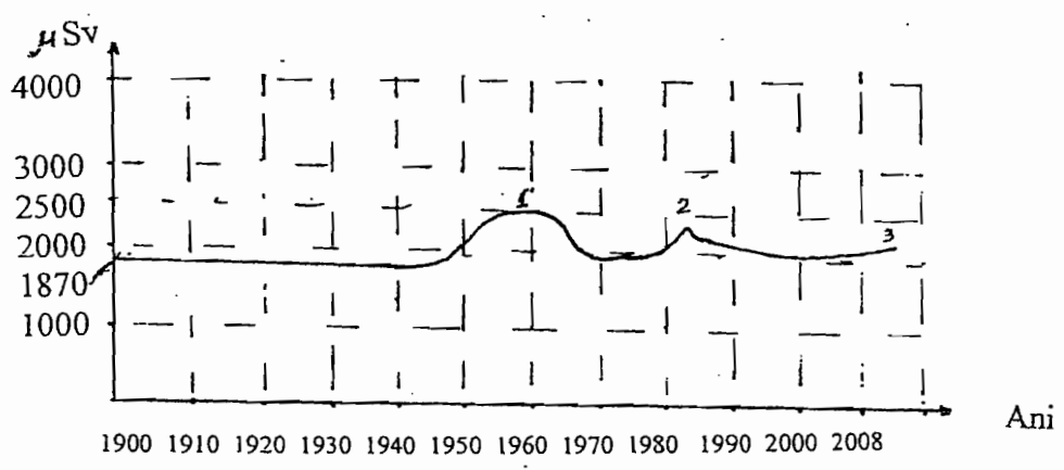
FIG. 2 EVOLUTIA RADIOACTIVITATII IN ATMOSFERA TEREI / OM / AN
