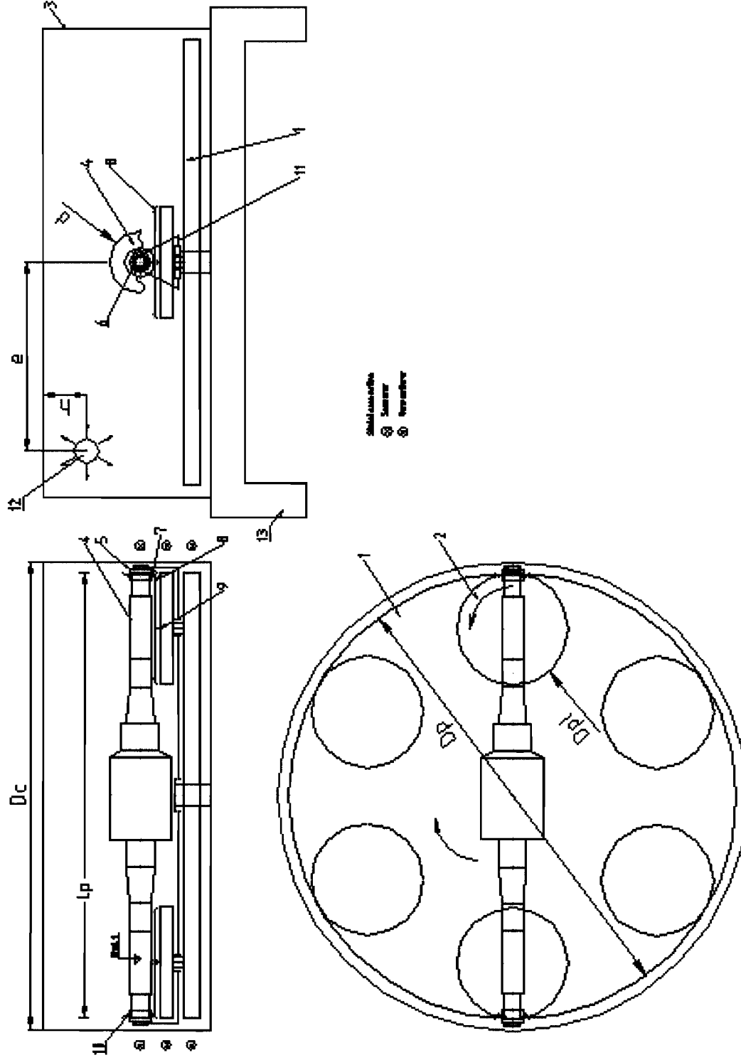
Fig.1 Dispozitiv pentru expunere spatiala a pieselor, cu dimensiuni maxime, supuse emisiei ionilor de titan, in batiscaful instalatiei de titanizare, cu procesarea unei singure piese tip ax
